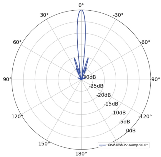
Port 2
